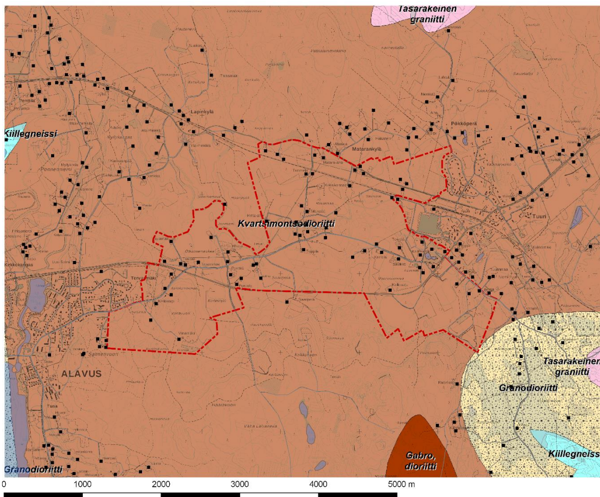
Kuva 2. Selvitysalueen kallioperä.
