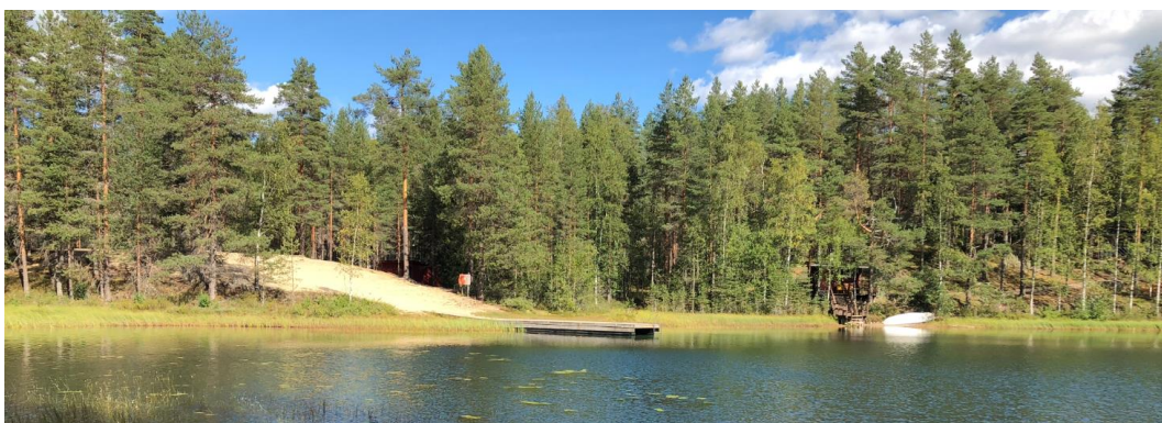
Kuva: 31 Valkeislammen pohjoisosan hiekkadyyni.
