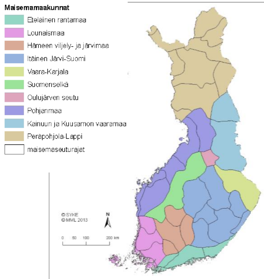
Kuva 1 Suomen maisemamaakuntajaossa Töysä sijaitsee Suomenselän ja Pohjanmaan rajalla. Kuva: SYKE & Maanmittauslaitos.
