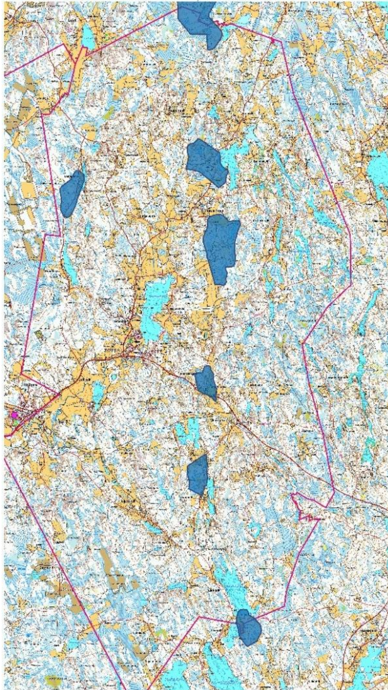
Kuva: 8 Ote alueen pohjavesialueista. Pohjakartta ©Maanmittauslaitos 06/2018 ja pohjavesitiedot Syke avoin aineisto.
