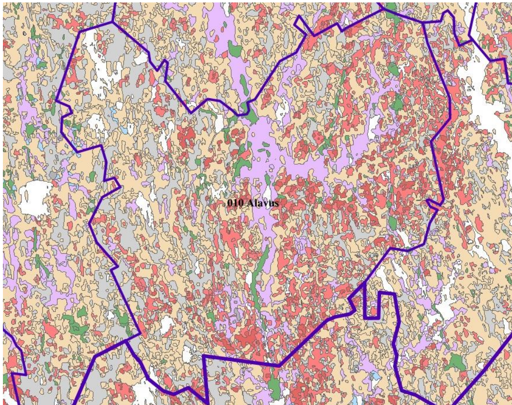
Kuva: 7 Ote maaperäkartasta. Lähde: paikkatietoikkuna 08/2018.
